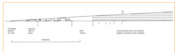
Figure 10 Section de la ligne de visée ascendante depuis le pont de St. James's Park sur Duck Island avec Downing Street au-delà.
